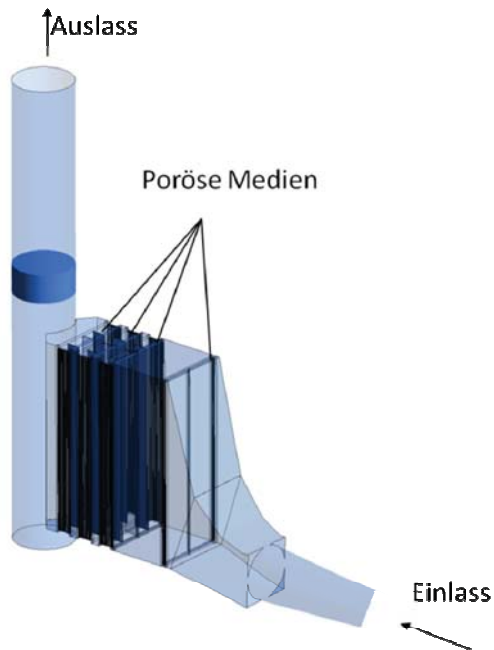
Abb. 8: Randbedingungen der Strömungssimulation: Am Einlass werden Geschwindigkeit und Temperatur, am Auslass der Druck vorgegeben, alle übrigen Ränder sind adiabatische Wände. Die porösen Medien modellieren Impuls- und Wärmeabgabe an die Wärmetauscherrohre.
