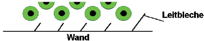
Abb. 3: Prinzipskizze der Leitbleche und Wärmetauscherrohre an der Wand; die Leitbleche sollen den Bypass verringern.
