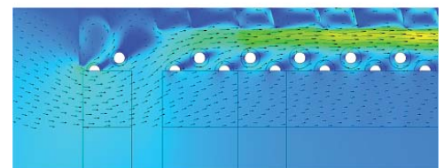
Geschwindigkeit im Bypass zwischen Rohrpaket und Leitbleche (Bild: CFX Berlin Software GmbH)
